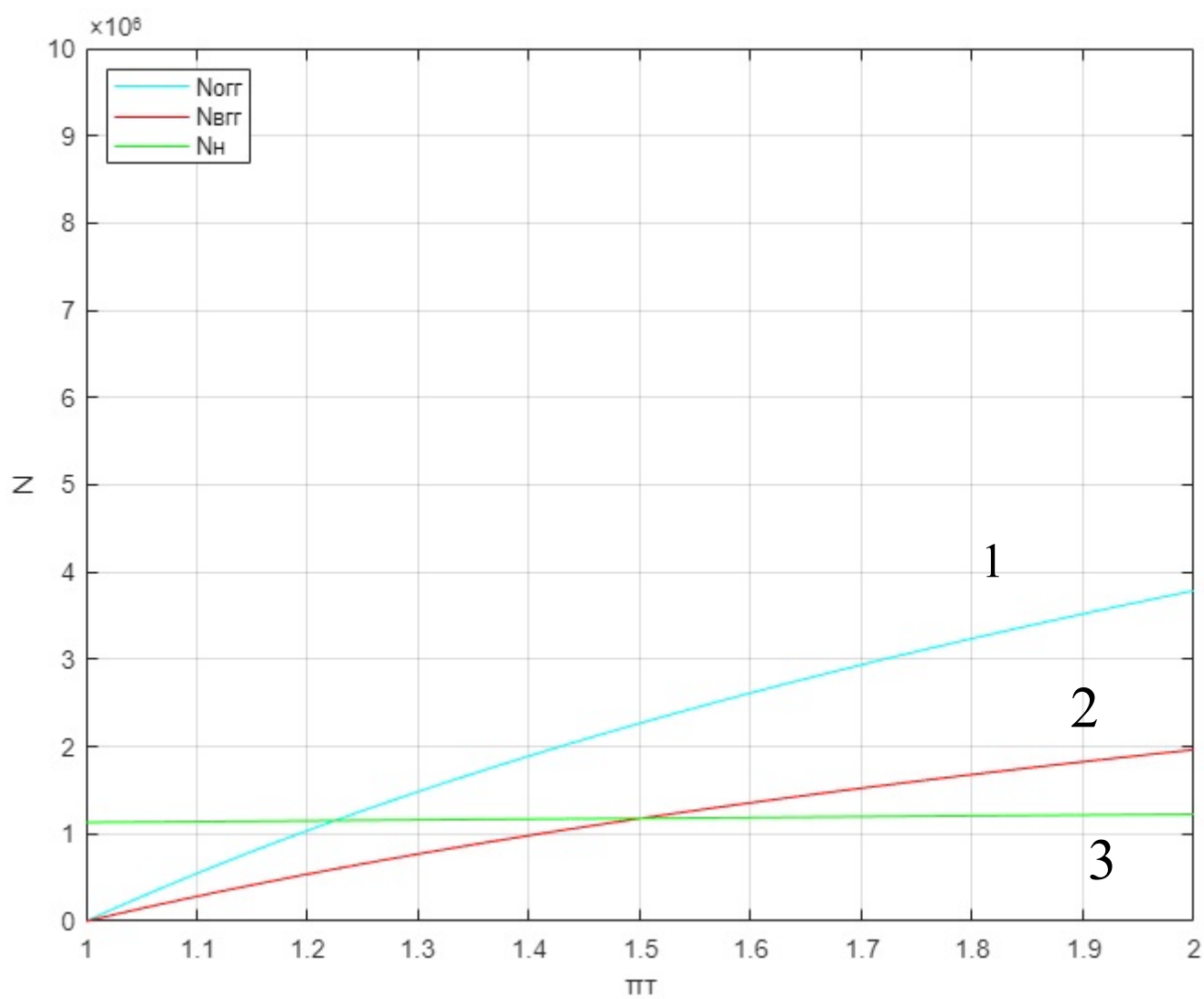
Рис. 1. К решению задачи: 1 — N_{т.ок} при окислительном ЖГГ; 2 — N_{т.гор} при восстановительном ЖГГ; 3 — N_{н}
